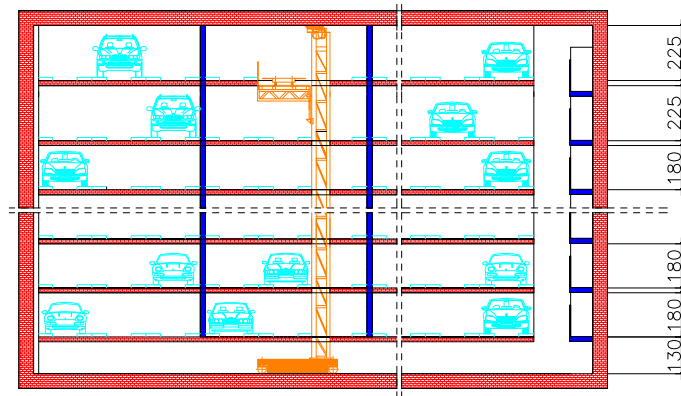
Cross section A-A Τομή A-A
