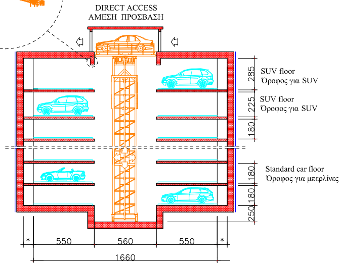
Cross section B-B Τομή B-B
