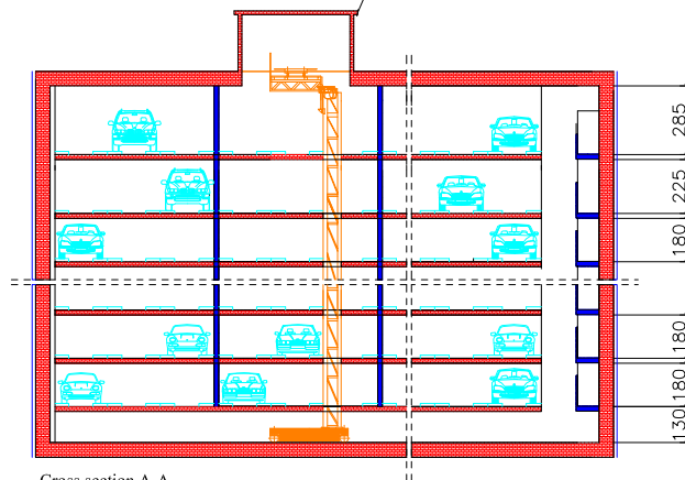
Cross section A-A Τομή A-A
