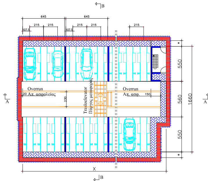
Typical floor plan Τυπικός όροφος
